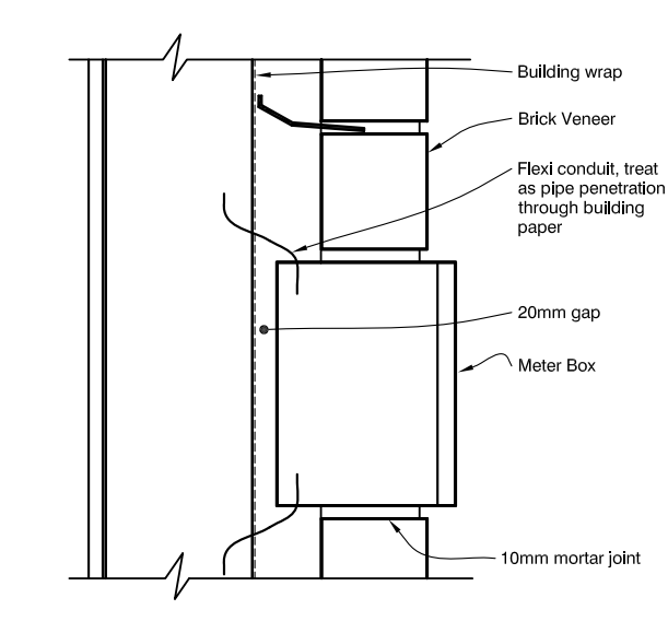
FIG.17 METER BOX
